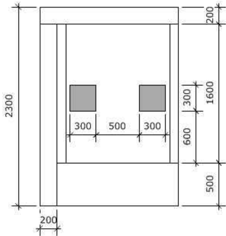
4 Internal Elevation Scale: 1:25
