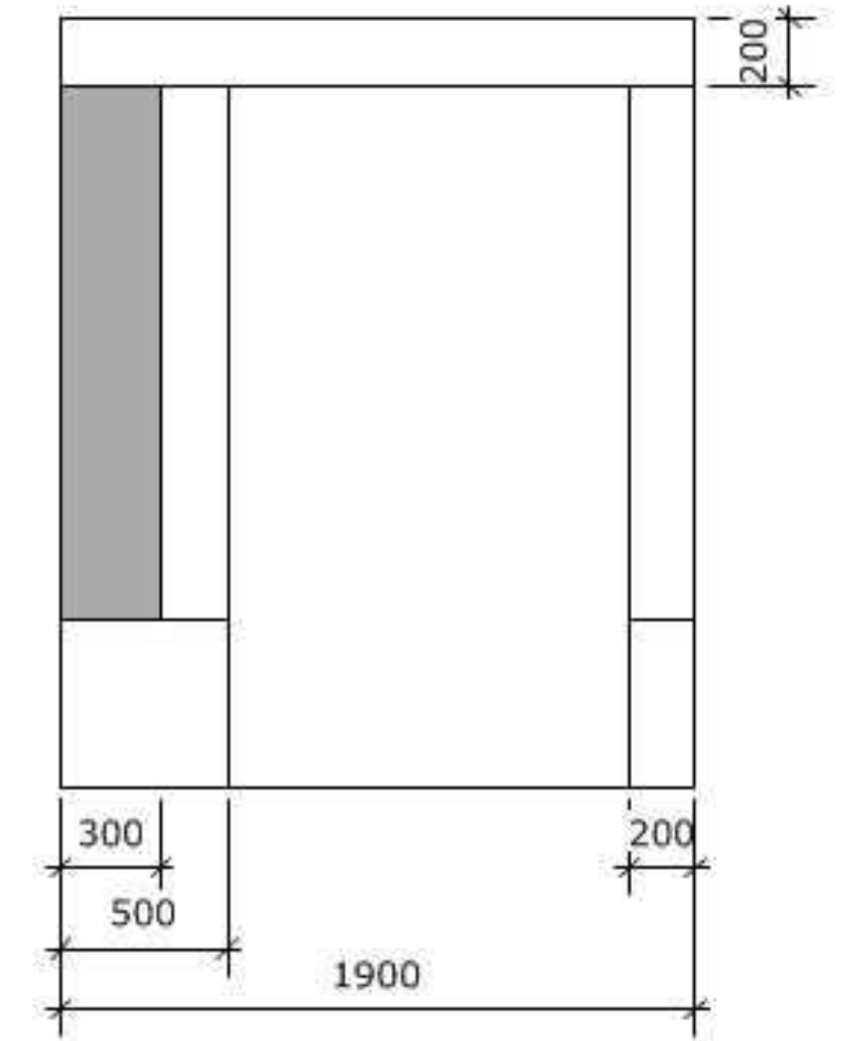
3 External Elevation Scale: 1:25
