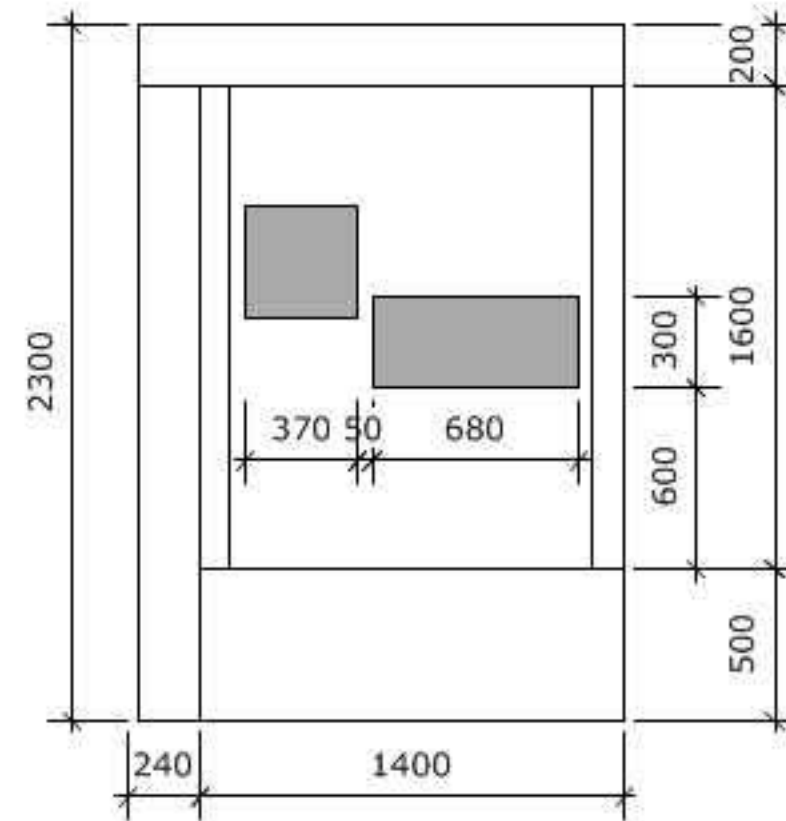
5 Internal Elevation Scale: 1:25
