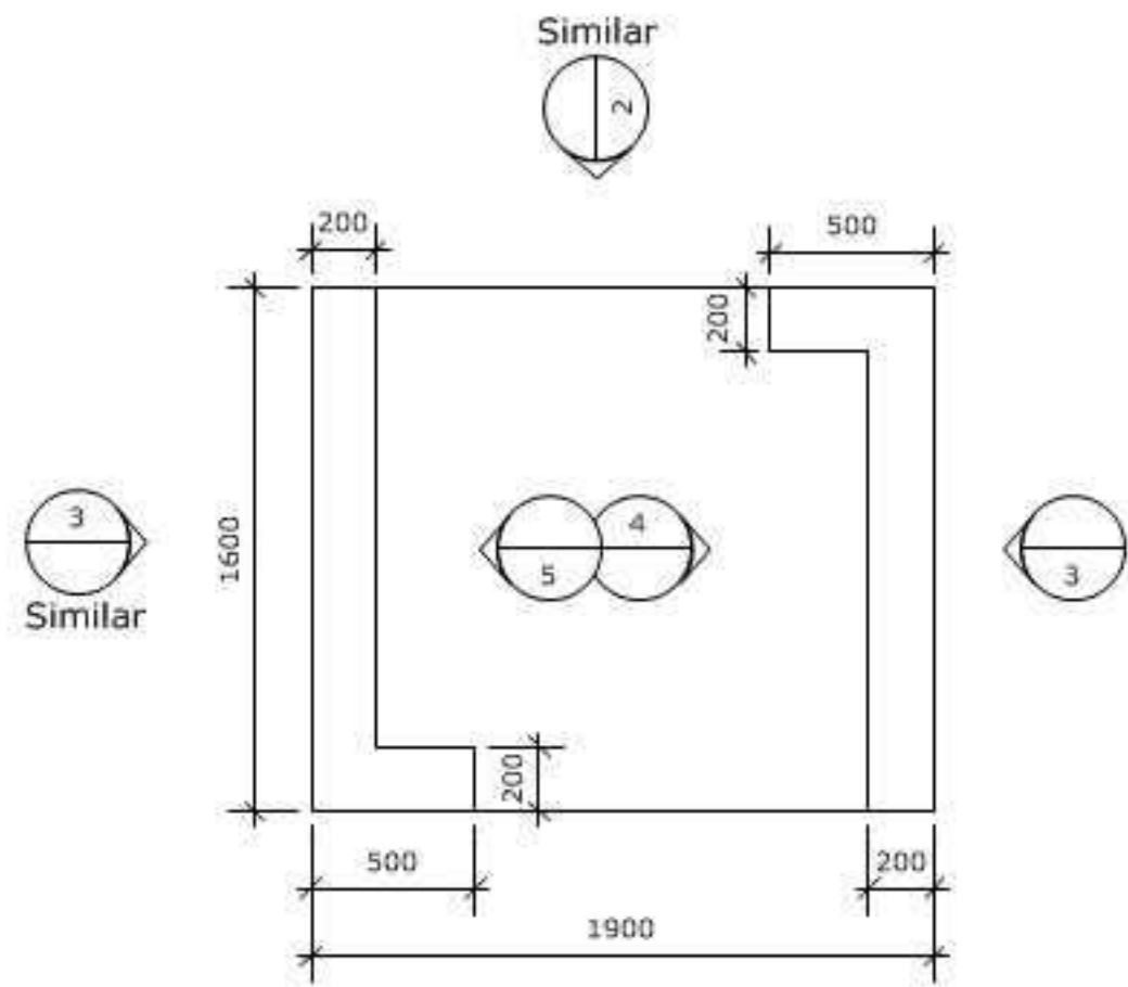
1 Plan Scale: 1:25
