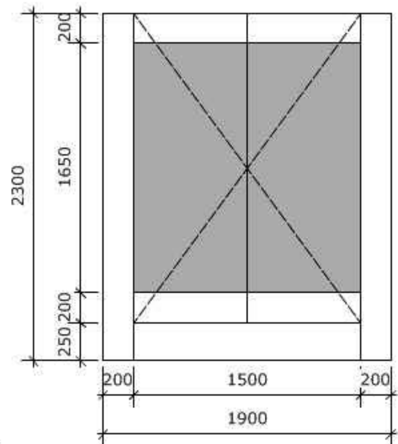
2 External Elevation Scale: 1:25
