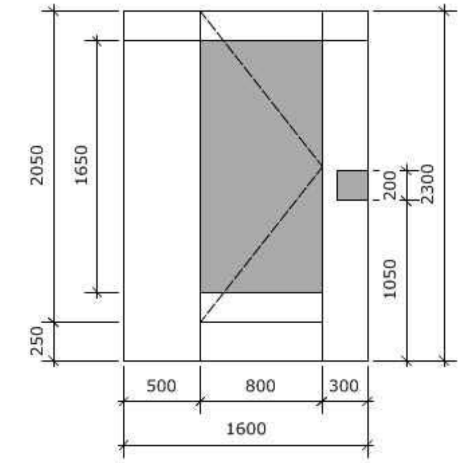
3 External Elevation Scale: 1:25
